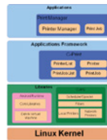
Android印刷フレームワーク
